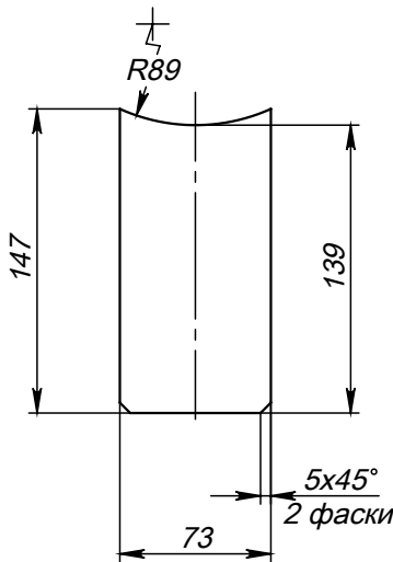
Поз.3 (Ребро)
