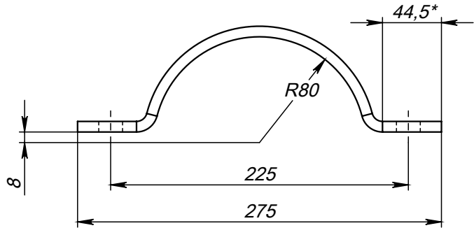
Поз.4 (Полухомут)
